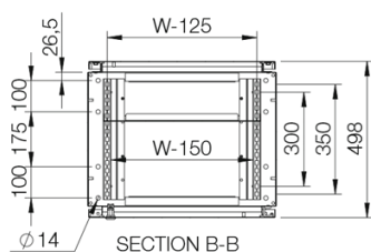
Double door
