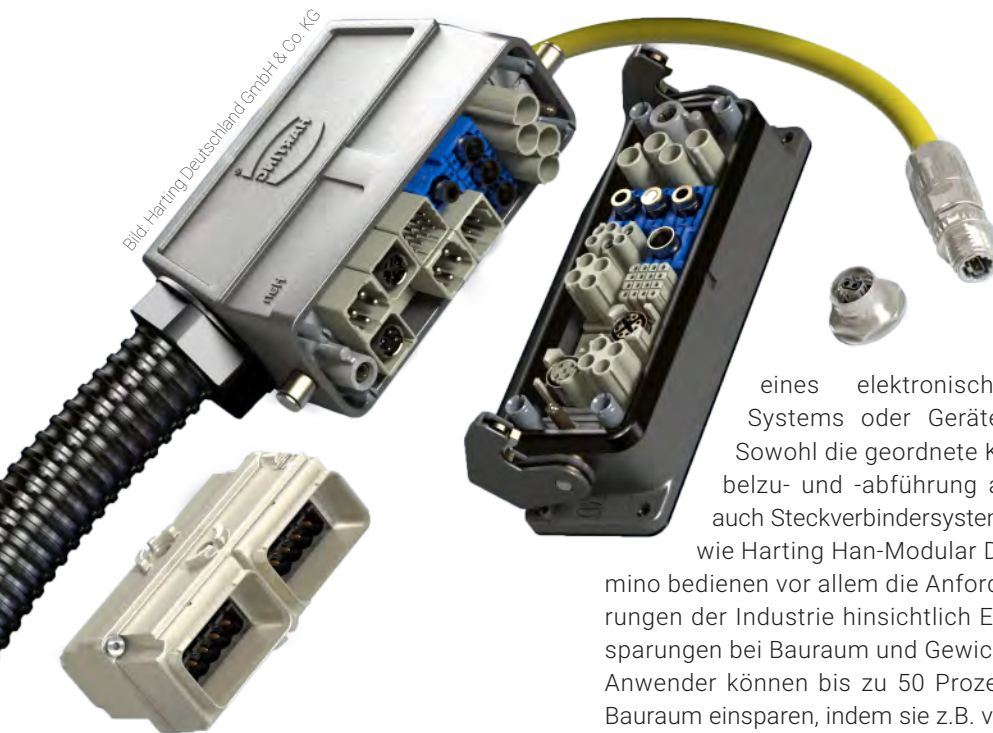
Bild 4 | Han-Modular Domino Module – mehr Platz, weniger Gewicht
