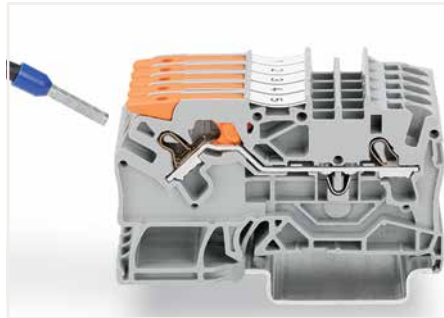
Direktes Stecken (Push-in) – feindrängige Leiter mit Aderndhülse
