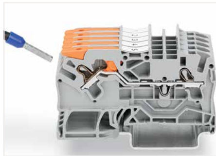
Direktes Stecken (Push-in) – feindrängige Leiter mit Aderndhülle
