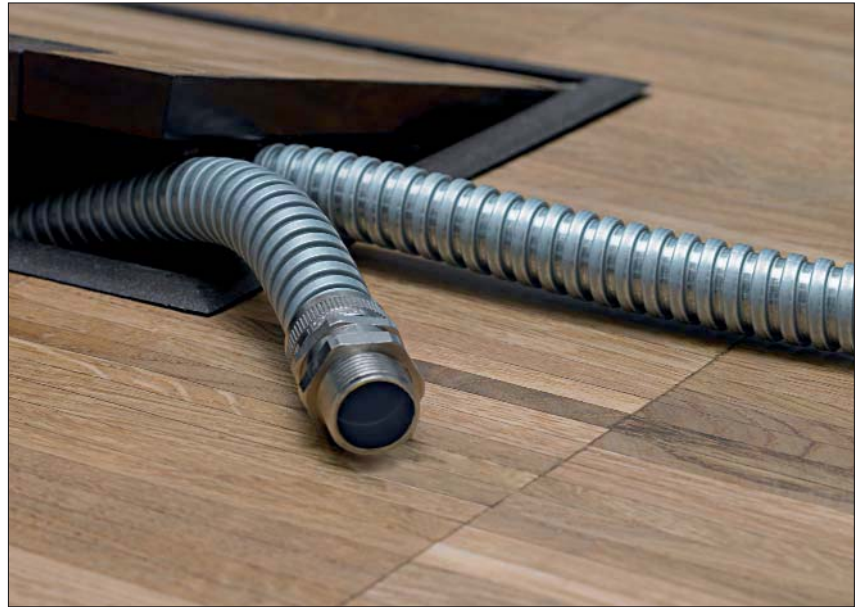
HelaGuard SC, galvanisierter Stahl-Schutzschlauch.
