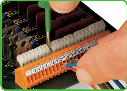
Leiter anschließen/lösen.
