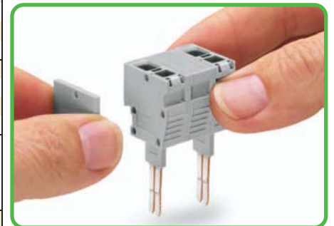
Zusammenrasten von Prüfstecker- und Blindmodulen mit Distanzplatten zu mehrpoligen Prüfsteckerleisten (max. 10-polig).
